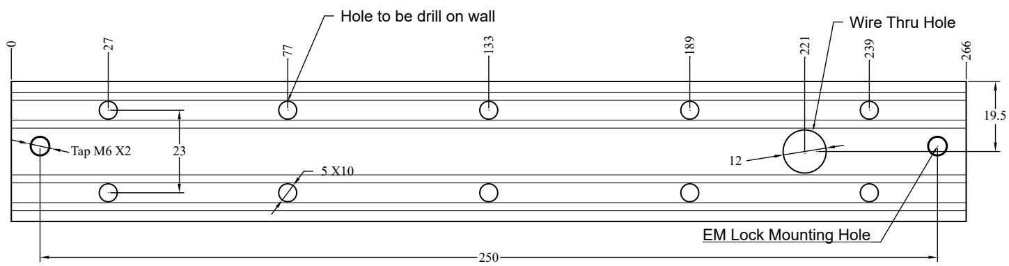
EM Lock Mounting Template
